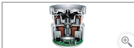
Moteur à impulsion numérique
